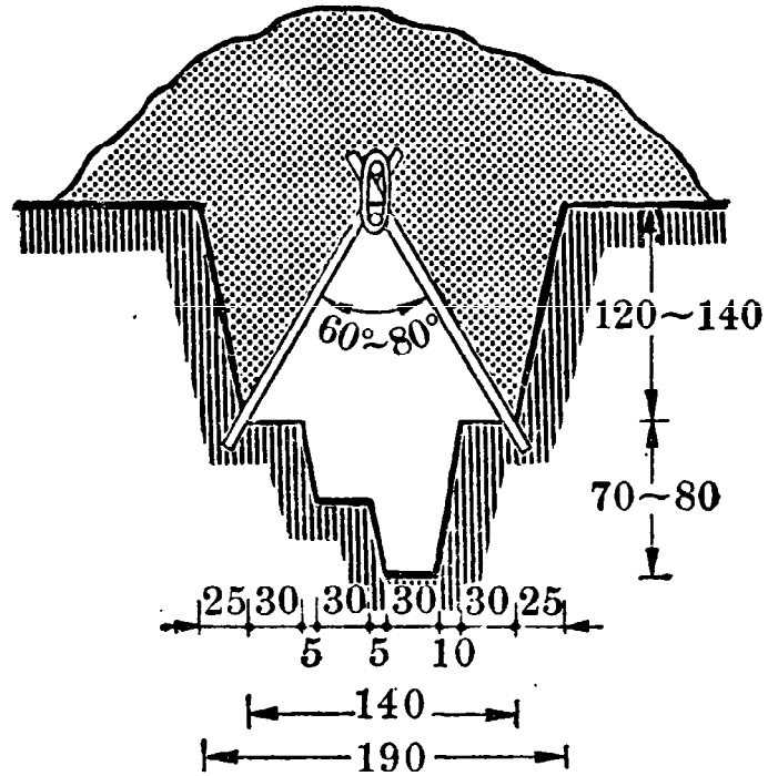
图 3-107 人字形骨架避弹所
