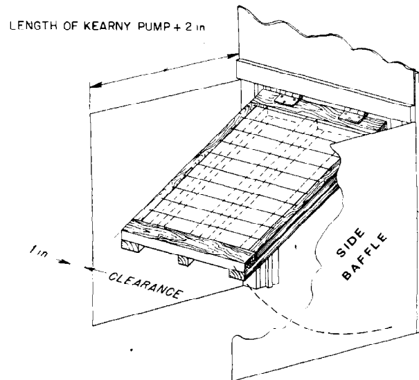
Fig. 25. Side baffles.
